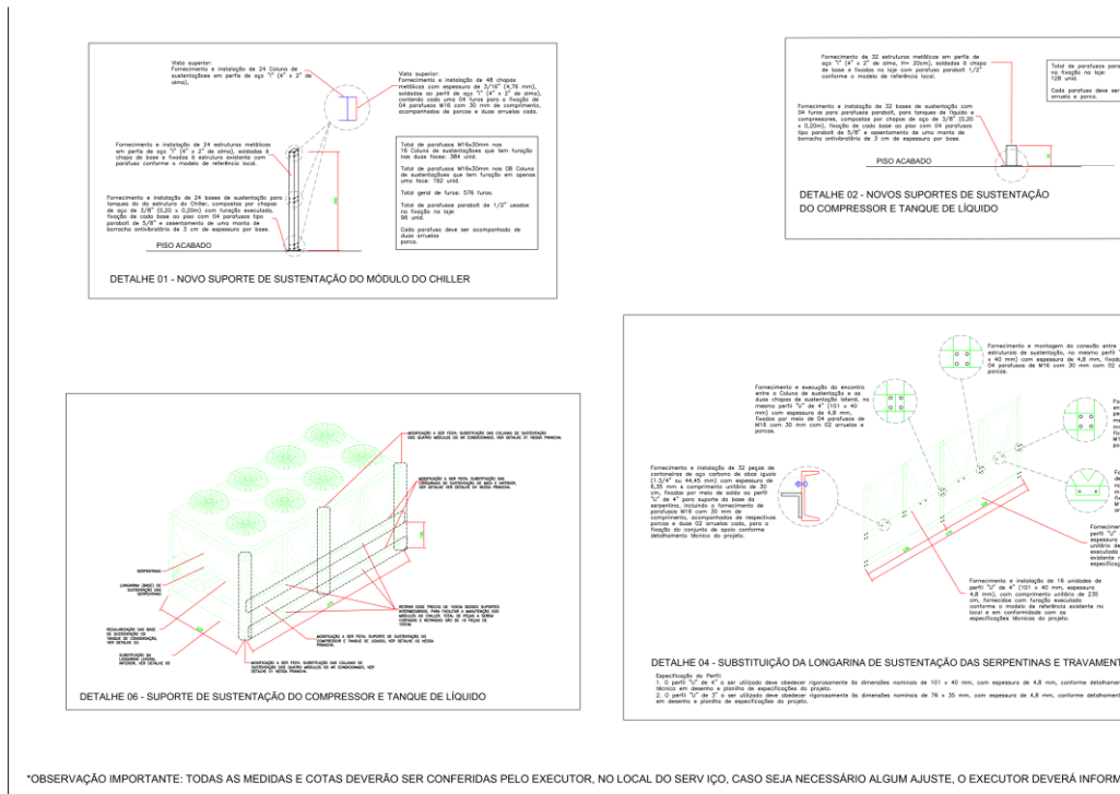
Figura 1: Detalhe Executivo do Carrinho e Suportes de Elevação da CAG
